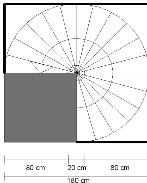
escalier accessoire
